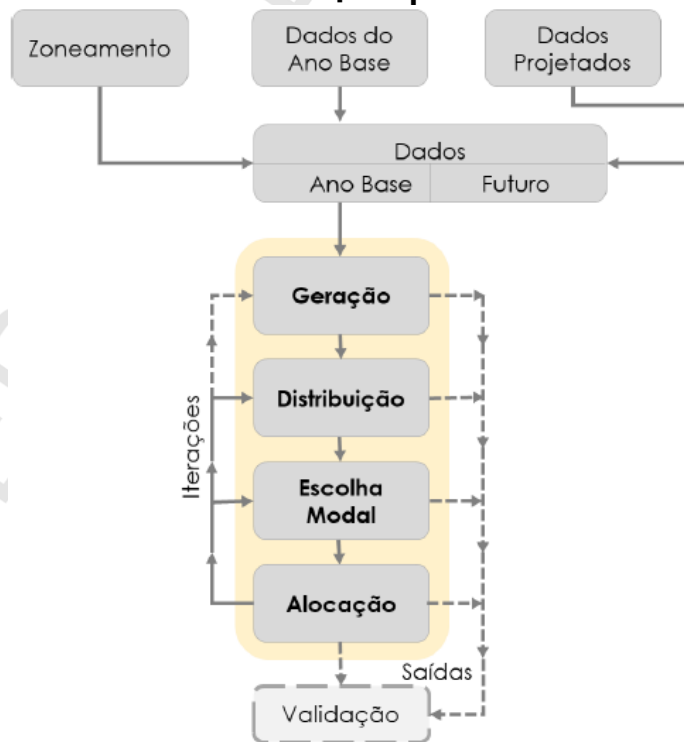
Figura 7 - Processo do modelo de 4 etapas
